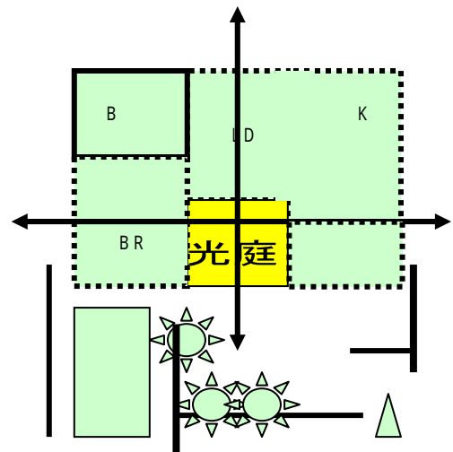
ダイレクトゲイン
